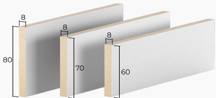
ГРУНТОВАНИЙ МДФ, ВИСОТОЮ 60, 70 або 80мм
