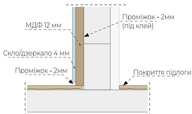
СТИКУВАННЯ ПАНЕЛІ ДО ПІДЛОГИ
