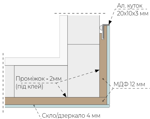
КУТОВЕ СТИКУВАННЯ ПАНЕЛЕЙ
