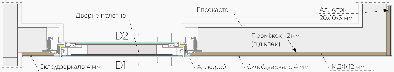
ВНУТРІШНЄ ВІДКРИВАННЯ ПОЛОТНА
